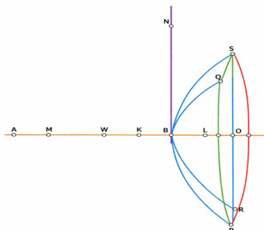
Рис. 2. Геометрическая схема построения линзы у Ибн Сахла, предназначенной для фокусировки параллельных солнечных лучей в конечной точке: точки A, B, K, L, M, N, O, S, R и P задают основные элементы построения, а вращение дуги гиперболы вокруг оси AB образует гиперboloидальную преломляющую поверхность, обеспечивающую сходимость преломлённых лучей в точке A.
