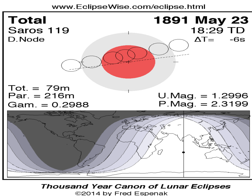
Рисунок 2. Схема полного лунного затмения 23 мая 1891 г. (Saros 119) и карта его географической видимости.
